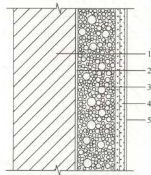
图 6.2.1 胶粉聚苯颗粒保温浆料外保温系统 1—基层墙体; 2—界面砂浆; 3—保温浆料; 4—抹面胶浆复合玻纤网; 5—饰面层
