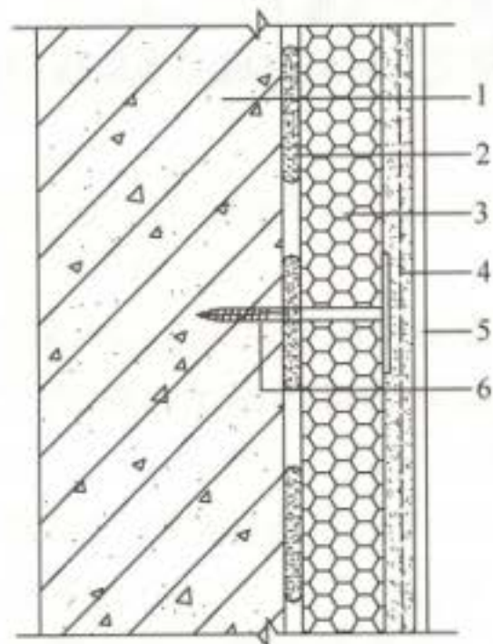
图 6.1.1 粘贴保温板薄抹灰外保温系统 1—基层墙体; 2—胶粘剂; 3—保温板; 4—抹面胶浆复合玻纤网; 5—饰面层; 6—锚栓
