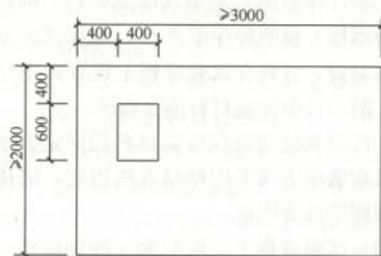
图 A.2.1-1 试验墙板 (mm)
