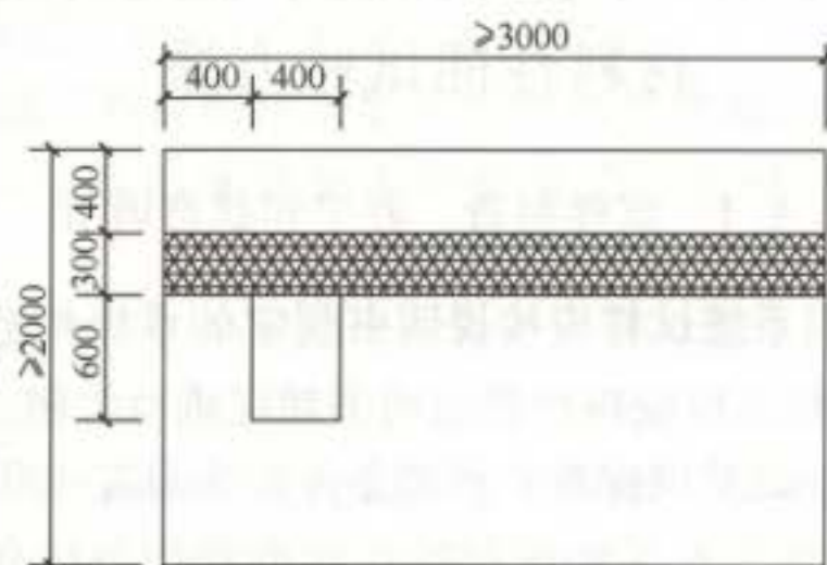
图 A. 2. 1-2 带防火隔离带试验墙板 (mm)
