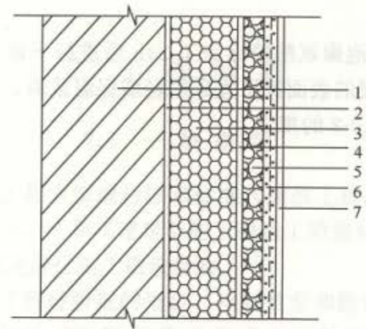
图 6.6.1 现场喷涂硬泡聚氨酯外保温系统
