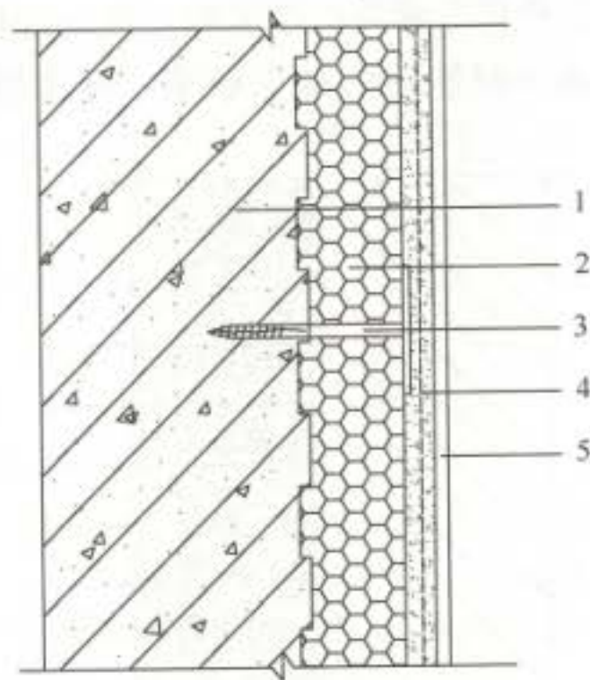
图 6.3.1 EPS板现浇混凝土外保温系统 1—现浇混凝土外墙；2—EPS板；3—辅助固定件； 4—抹面胶浆复合玻纤网；5—饰面层
