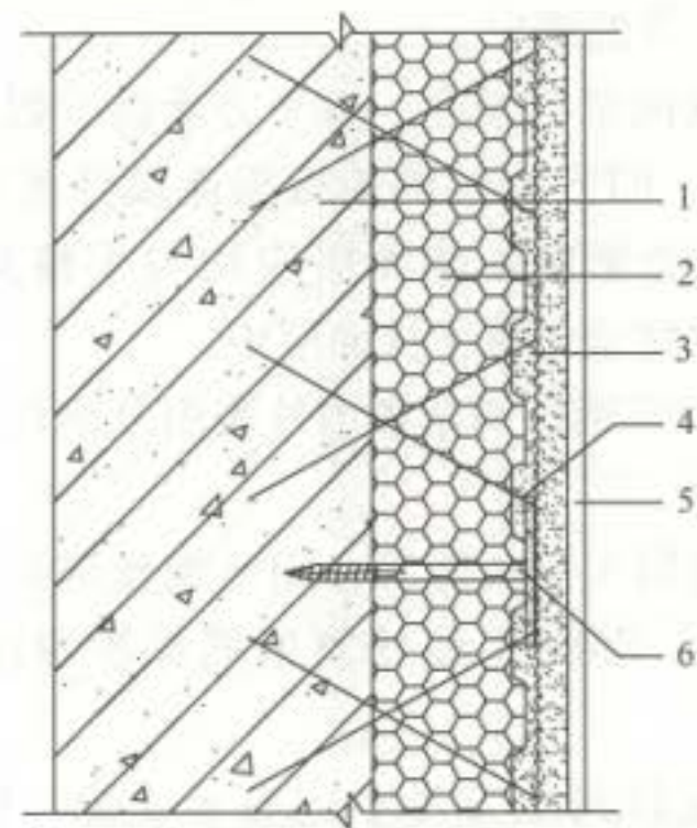
图 6.4.1 EPS钢丝网架板现浇混凝土外保温系统 1—现浇混凝土外墙；2—EPS钢丝网架板；3—掺外加剂的水 泥砂浆抹面层；4—钢丝网架；5—饰面层；6—辅助固定件
